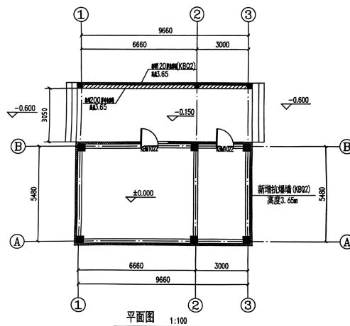
平面图 1:100
