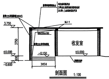
剖面图 1:100
