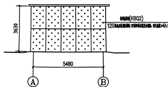
抗爆墙立面图 1:100
